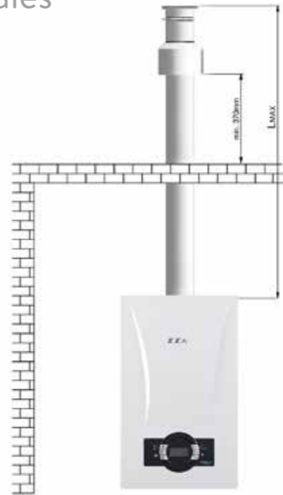
Aplicación de conductos de humos herméticos verticales L máx. distancia sin codo: 10 m, Ø60/100 L máx. distancia sin codo: 20 m, Ø80/125
